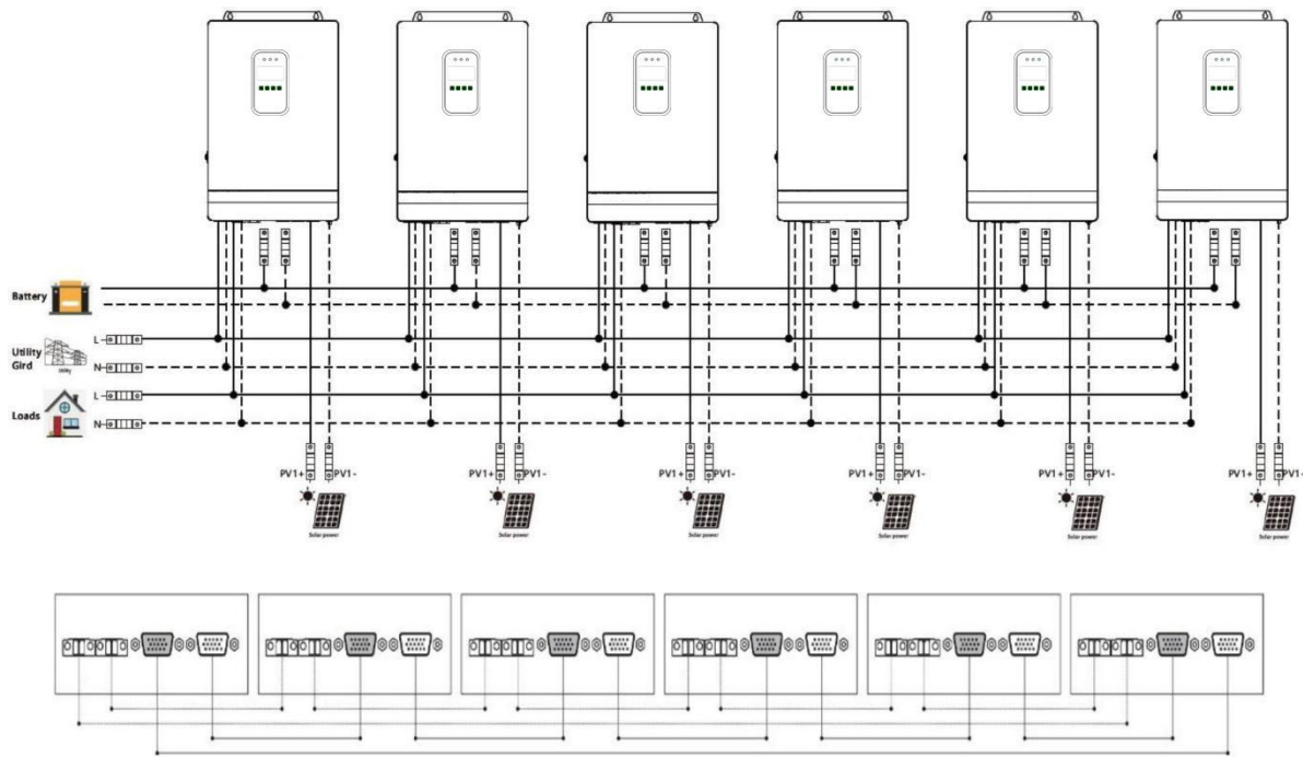
e) 系统六台逆控一体机并联：
