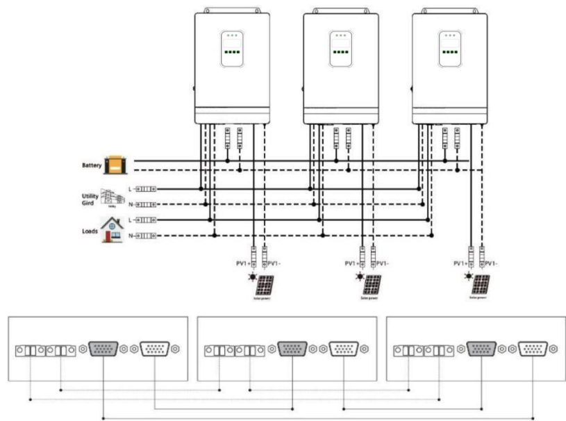
b) 系统三台逆控一体机并联：
