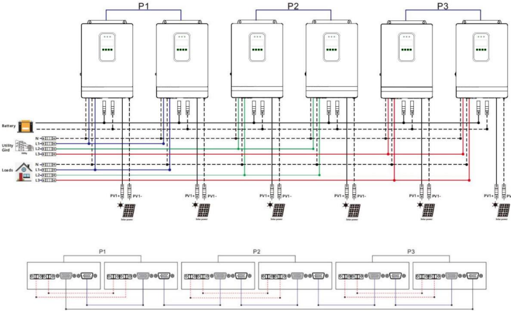
a) 六台设备组成三相相系统
