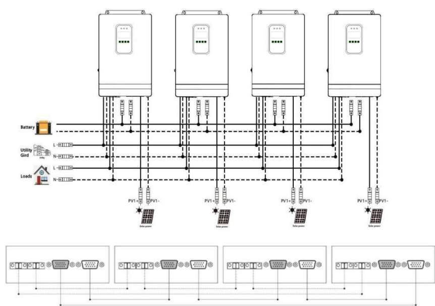
c) 系统四台逆控一体机并联：
